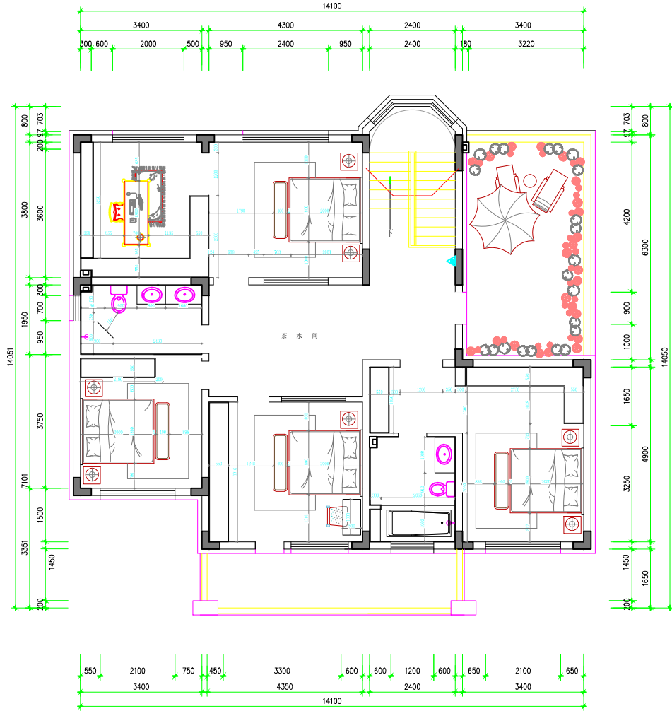
11#楼二层平面图 1:50
